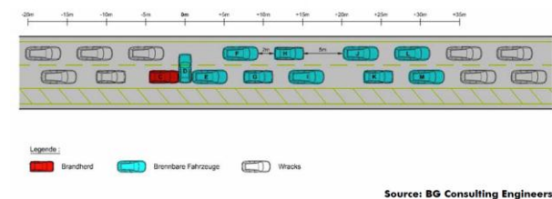
Abbildung 6: Grundriss des Versuchsaufbaus der A86-Brandversuche im Versuchsstollen Hagerbach
