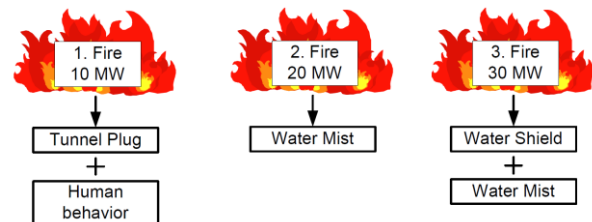
Abbildung 8: Versuchsprogramm im Virgolo-Tunnel 2005
