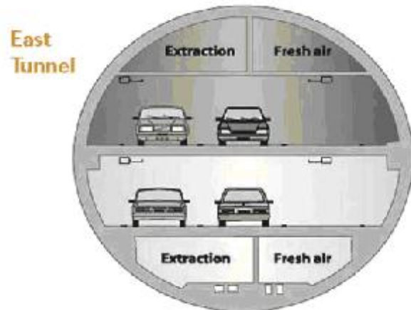
Abbildung 2: Lüftungssystem im A86-Tunnel ( http://www.fhwa.dot.gov/ )
