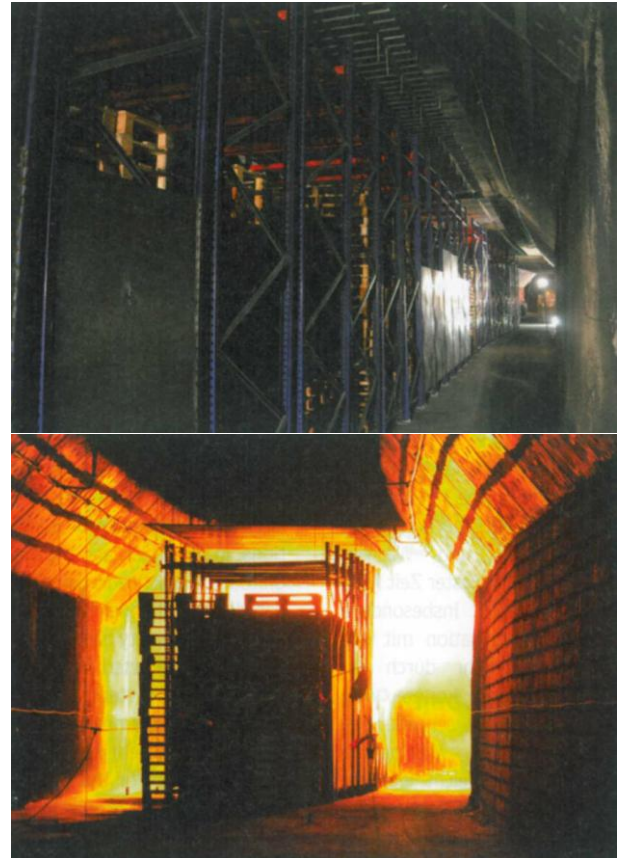
Abbildung 10: Versuchsaufbau und Brandversuch [Kratzmeir 2010]
