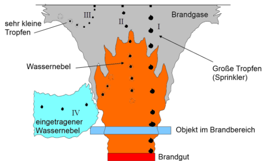
Abbildung 1: Wirkungsweise und -ort verschiedener Wassertropfengrößen [UPTUN 2006]
