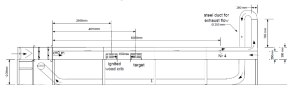
Abbildung 9: Schematische Darstellung des Versuchsaufbaus
