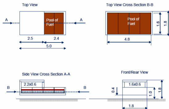
Abbildung 7: Brandlastwanne bei den UPTUN-Versuchen der DMT (2004) [UPTUN 2008a]
